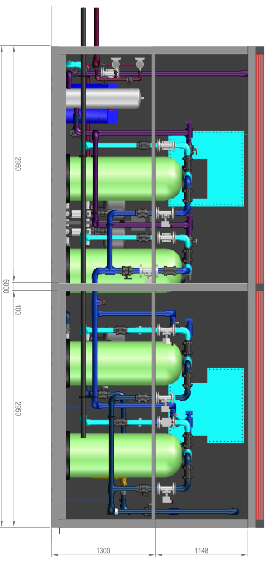
Вид А
